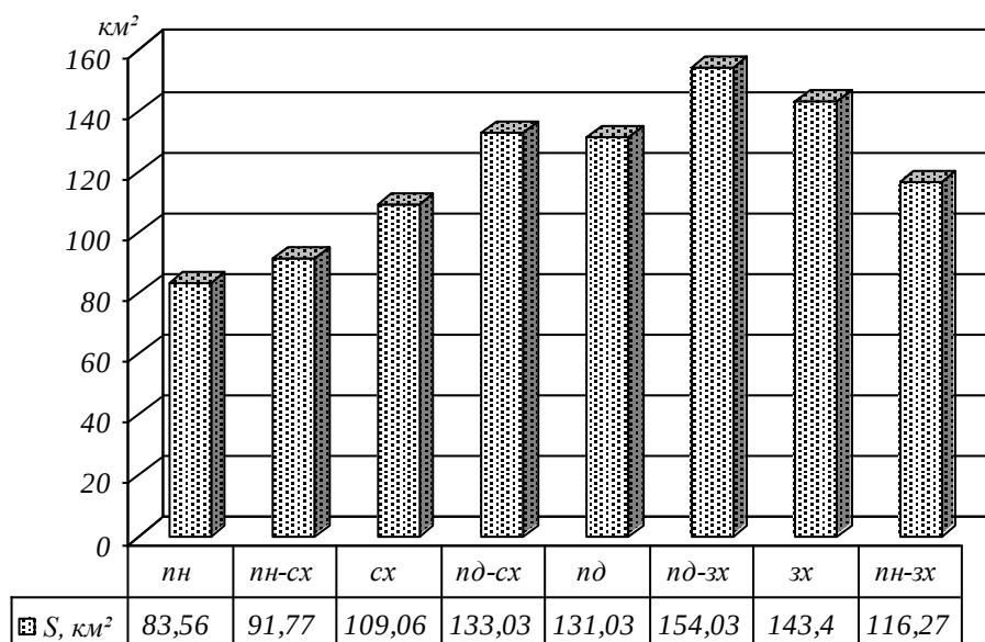
Рисунок 3. Експозиція схилів хребта Великий Діл
