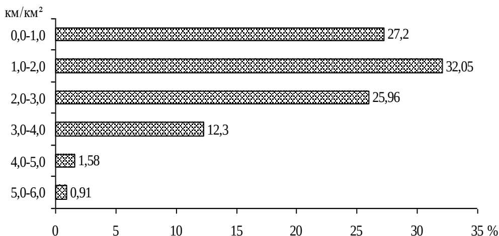
Рисунок 2. Горизонтальне розчленування хребта Великий Діл ( \text{км/км}^2 )
