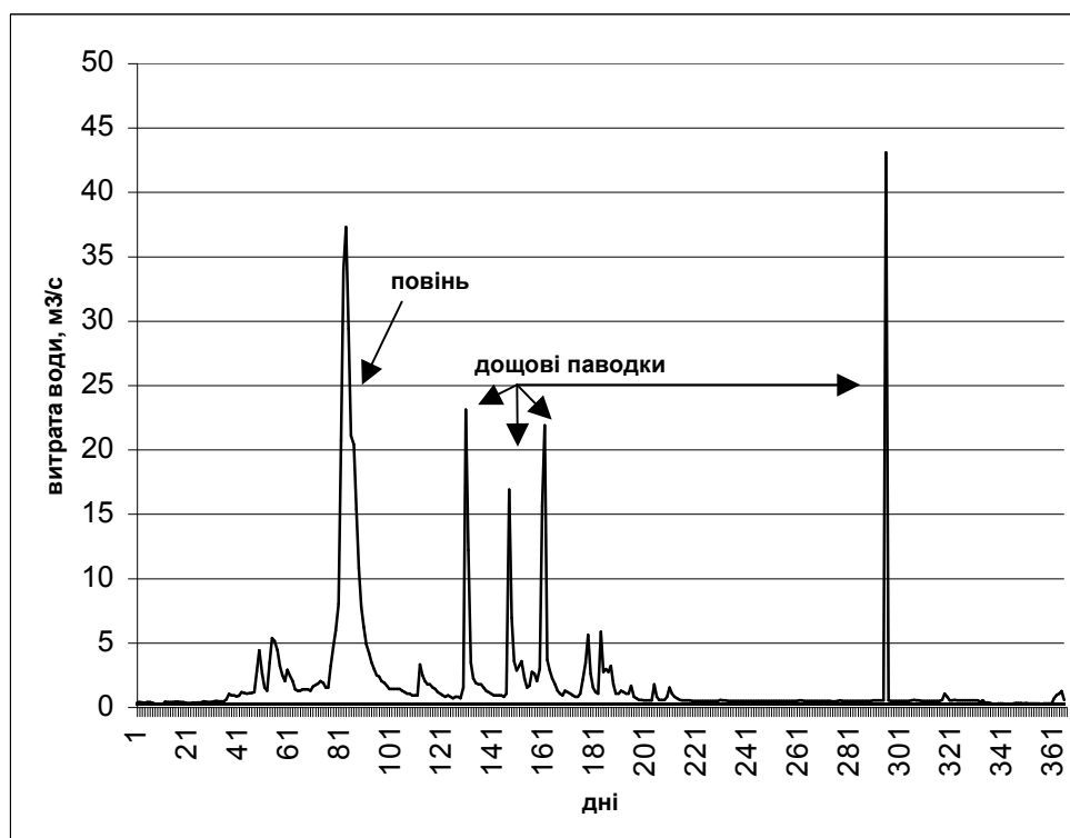
Рисунок 2. Річний хід витрат води на річці Дерелуй (1973 р.)
