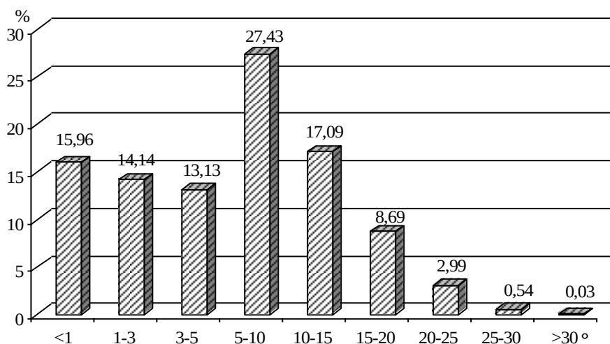
Рисунок 4. Крутість схилів хребта Великий Діл
