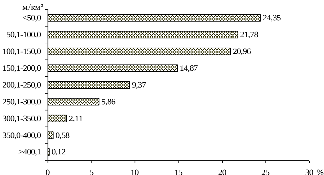
Рисунок 1. Вертикальне розчленування хребта Великий Діл (м/км 2 )
