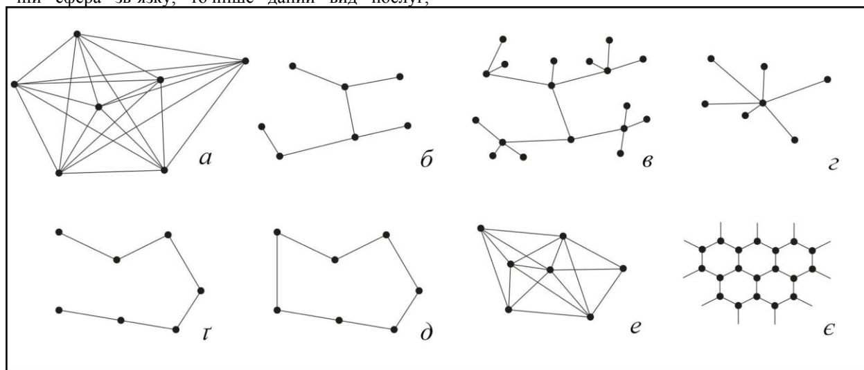
Рисунок 2. Види мереж зв'язку лінійно-вузлового типу:
